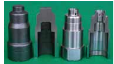
冷鍛一切削加工品の製品例
