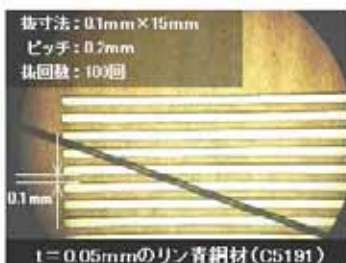
t=0.05mmのリン青鋼材(C5191)
