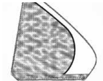
当社製品で測定した自動車ガラスの歪み分布
