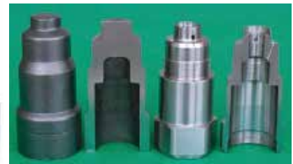
冷鍛一切削加工品の製品例
