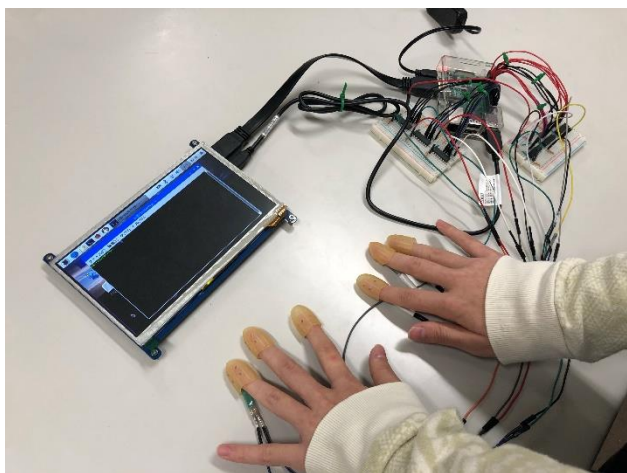
Raspberry Piを用いた指点字入出力装置
